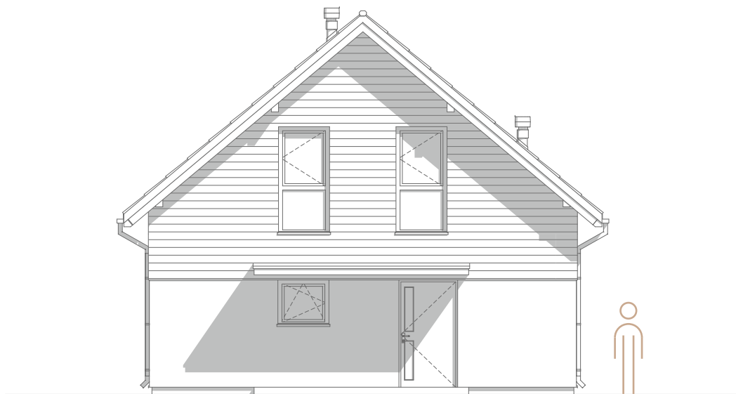
ELEWACJA 02
