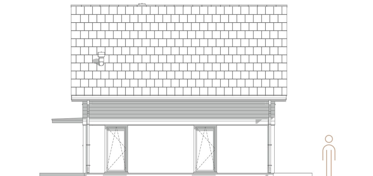
ELEWACJA 04
