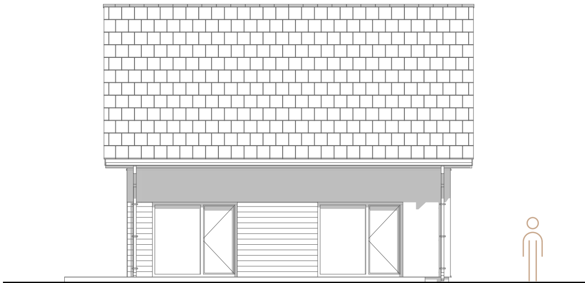
ELEWACJA BOCZNA 1
