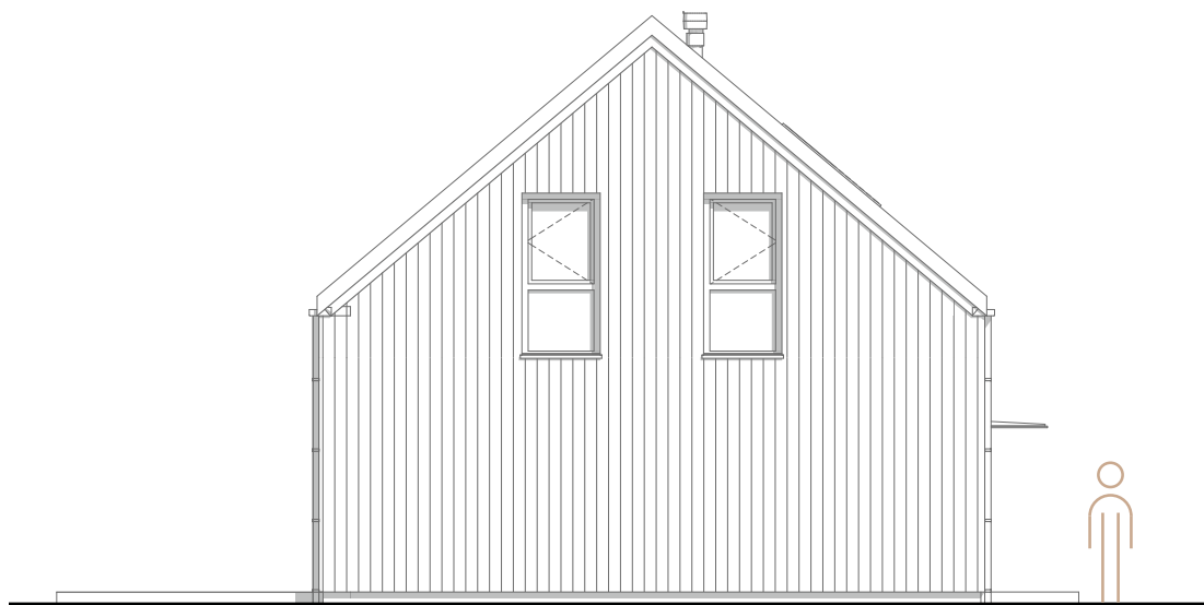
ELEWACJA BOCZNA 1
