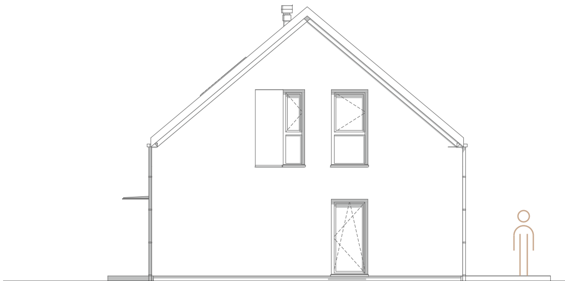
ELEWACJA BOCZNA 2
